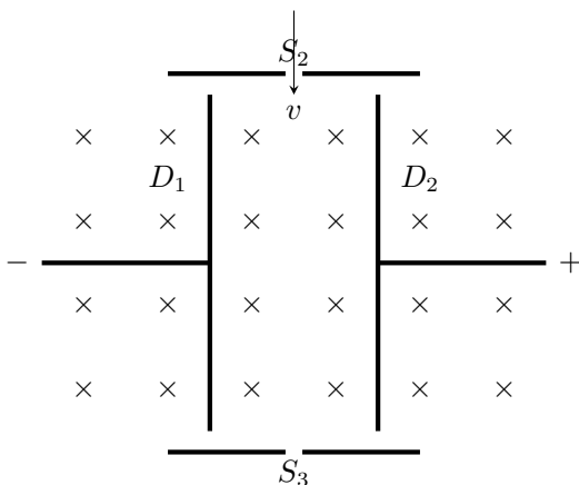
图 1.38 速度选择器的原理示意图
