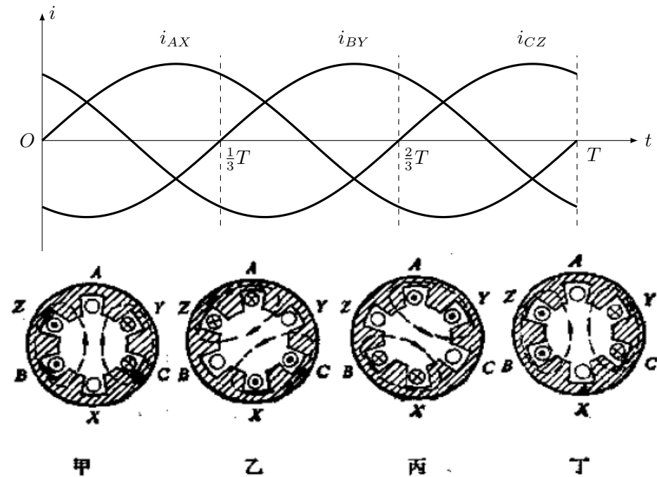
图 3.56 旋转磁场的产生
