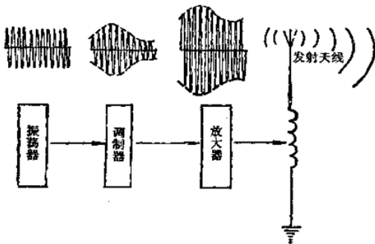
图 4.15 电磁波发送的方框图
