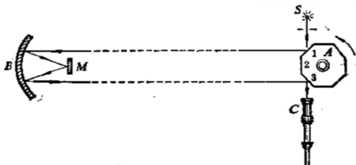
图 5.5 迈克耳孙测定光速实验的示意图
