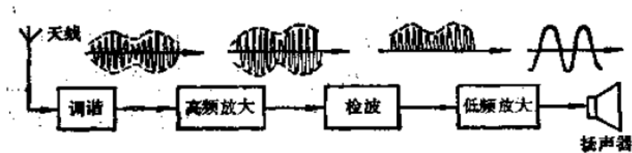
图 4.20 收音机的方框图
