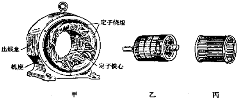
图 3.57 感应电动机的定子和转子
