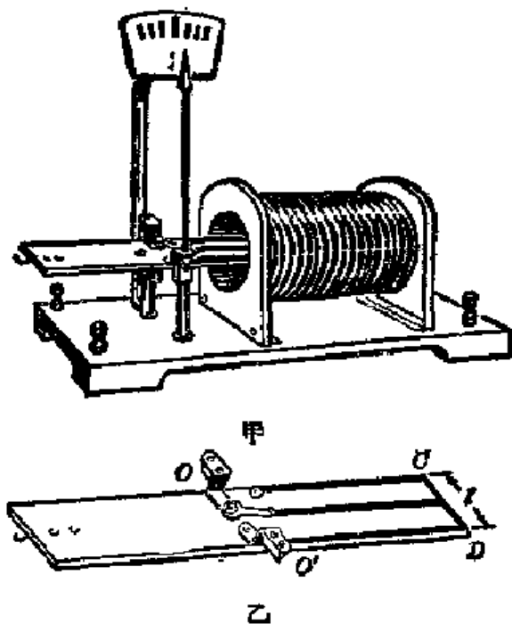
图 1.28 电流天平
