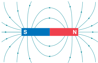
图 1.5 磁铁磁场的磁力线分布
