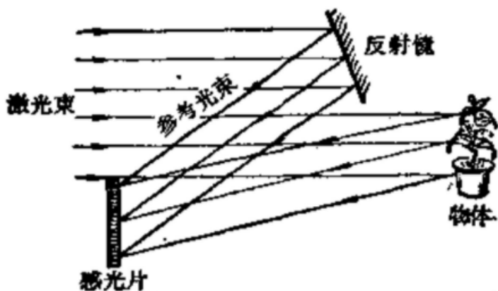
图 6.6 全息照相原理示意图
