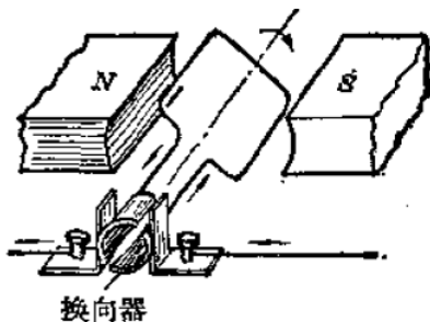
图 2.24 直流电动机的模型
