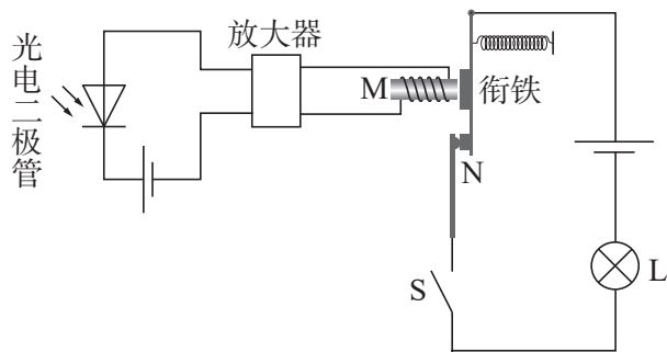
图 7.4 光控继电器示意图
