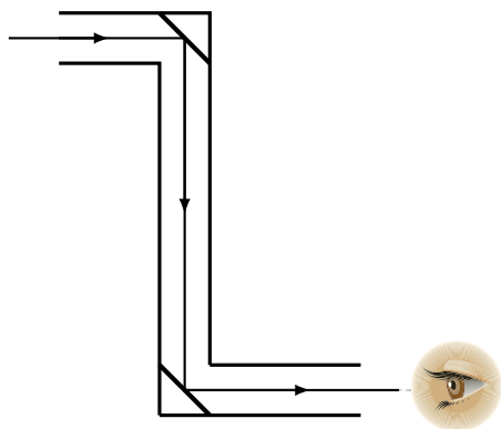
图 5.11 潜望镜示意图
