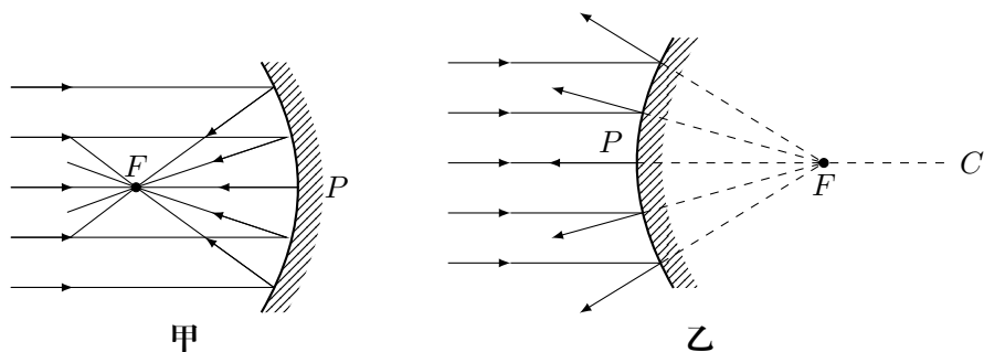
图 5.14 球面镜的焦点和焦距
