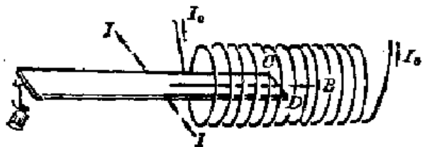
图 1.29 测定螺线管的磁感应强度
