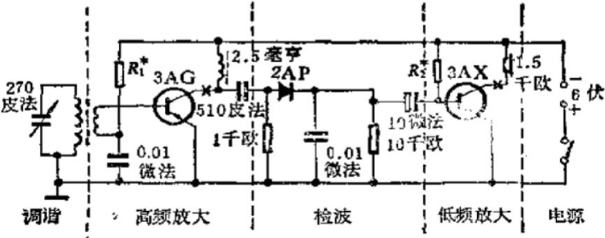
图 10.6 简单收音机的线路图
