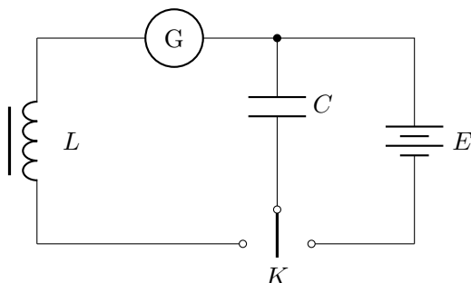
图 4.1 振荡电路
