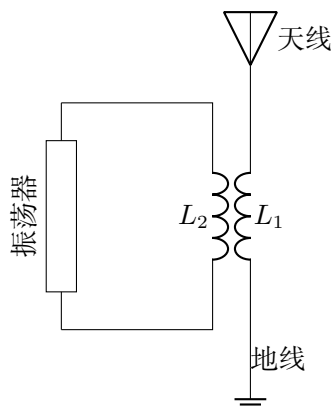
图 4.12 感应耦合
