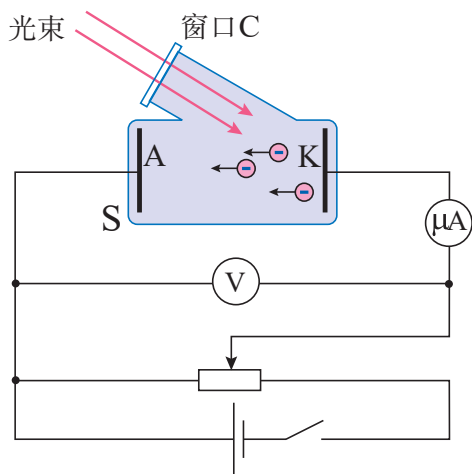
图 7.2 研究光电效应的装置简图
