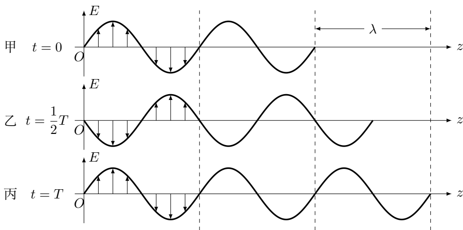
图 4.8 电磁波以一定速度在空间传播 (为简单起见只画出了 E 矢量)
