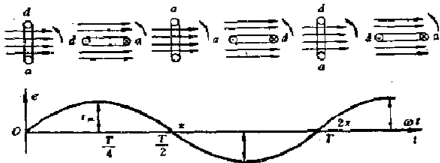
图 3.4 e = \mathcal{E}_m \sin \omega t 的图象
