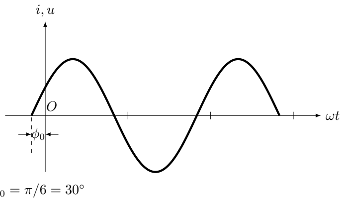
图 3.5 i = I_m \sin(\omega t + \phi_0) 或 u = U_m \sin(\omega t + \phi_0) 的图象
