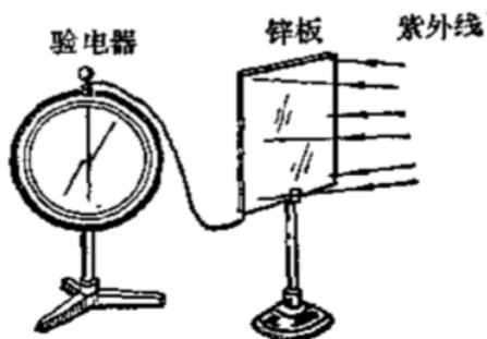
图 7.1 紫外线照射锌板使验电器带正电
