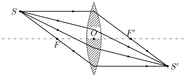
图 5.39 像是通过凸透镜的所有光线的会聚点
