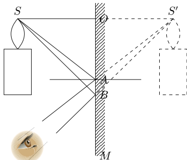
图 5.10 平面镜成虚像
