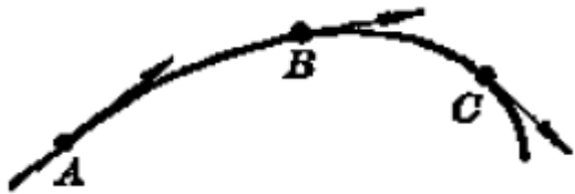
图 1.4 磁力线
