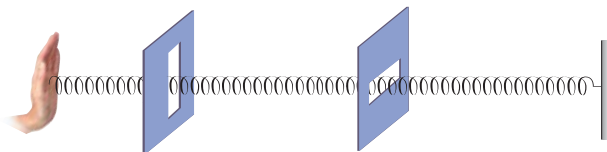
图 6.12 纵波没有偏振现象
