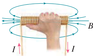
图 1.8 通电螺线管的磁场
