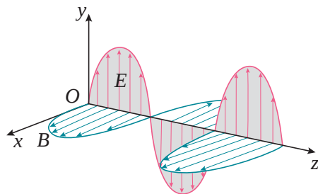
图 4.7 沿 z 轴传播的电磁波在某一时刻的波的图象
