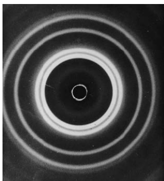
图 7.7 伦琴射线衍射图样
