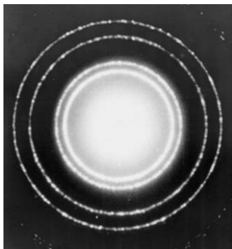
图 7.6 电子衍射图样
