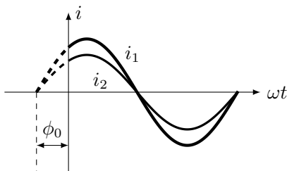
图 3.6 图中的 i_1 = I_m \sin(\omega t + \phi_0) , i_2 = I'_m \sin(\omega t + \phi_0)
