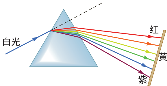
图 5.32 棱镜使白光发生色散
