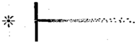
图 5.1 光沿直线传播
