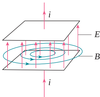
图 4.5 变化的电场产生磁场
