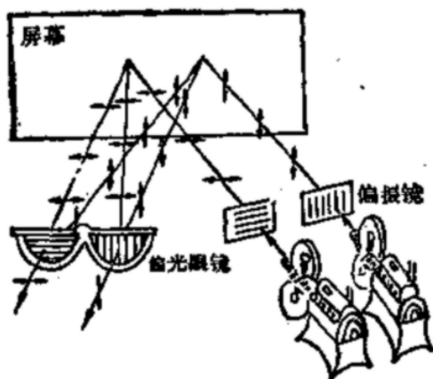
图 6.15 立体电影
