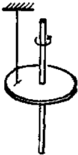
图 1.9 罗兰实验的示意图
