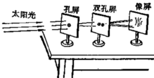
图 6.1 杨氏实验
