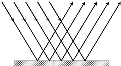
图 5.8 镜面反射
