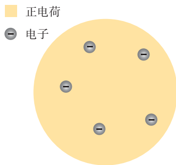
图 8.1 汤姆生的原子模型
