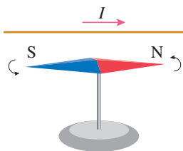
图 1.1 奥斯特实验
