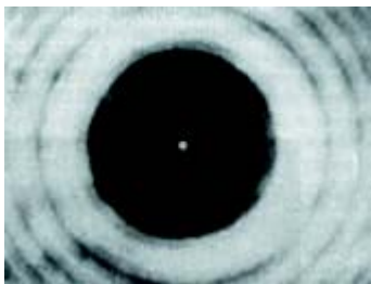
图 6.8 不透明盘产生的衍射，影子的中心有一个亮斑（泊松亮斑）
