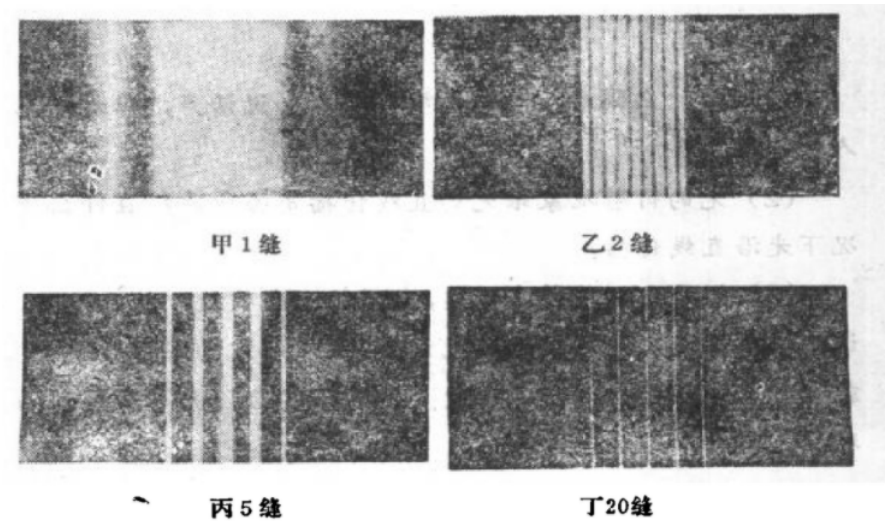
图 6.9 衍射条纹随着缝数增加而变窄
