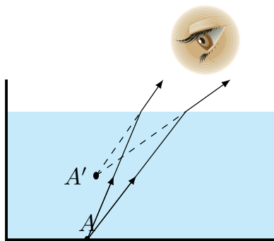
图 5.20 水的视深比实深浅
