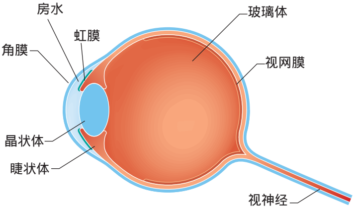
图 5.49 眼睛构造简图
