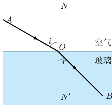
图 5.19 光从空气进入玻璃时发生折射
