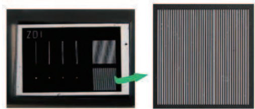
图 6.10 衍射光栅
