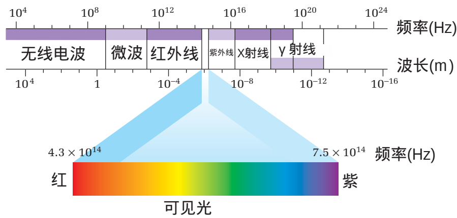
图 6.17 电磁波谱
