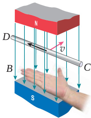
图 2.14 右手定则
