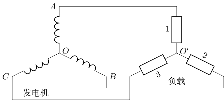
图 3.50 三相三线制
