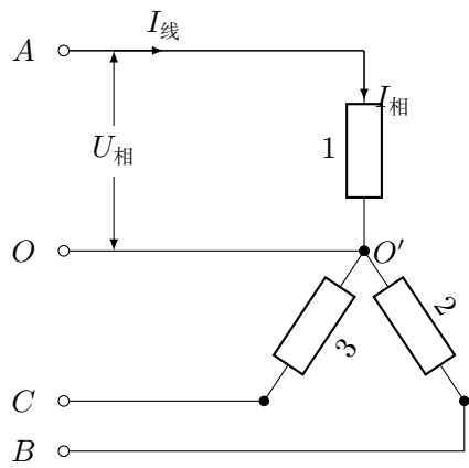
图 3.48 负载的星形连接
