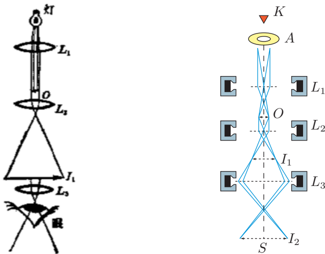
图 5.56 用磁场聚焦的电子显微镜的示意图 (右图)
