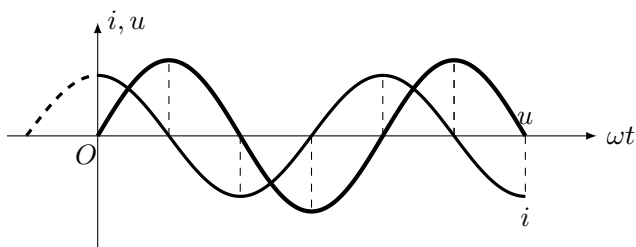
图 3.22 电容对交流电相位的影响
