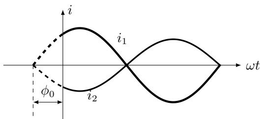
图 3.7 图中的 i_1 = I_m \sin(\omega t + \phi_0) , i_2 = I'_m \sin(\omega t + \phi_0 + \pi)
