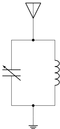
图 4.17 调谐电路
