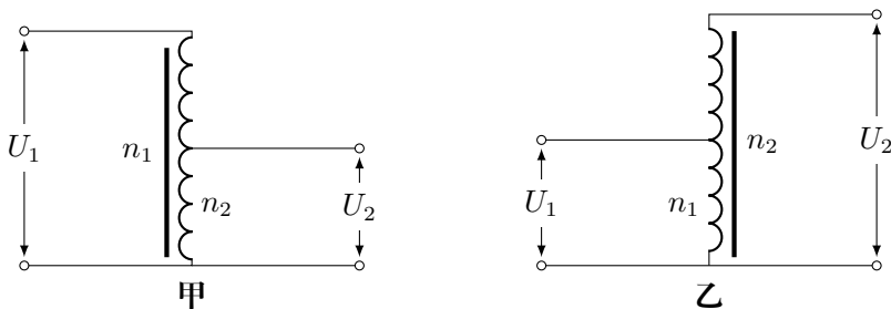
图 3.26 自耦变压器
