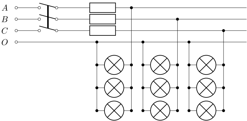
图 3.46 三相四线制中灯泡的连接
