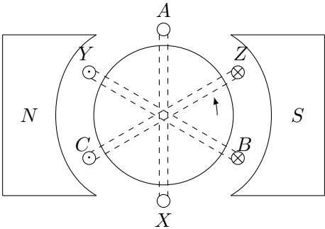
图 3.42 三相发电机的示意图
