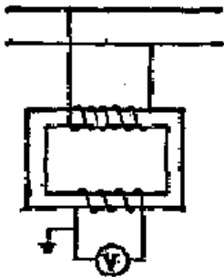
图 3.28 电压互感器
