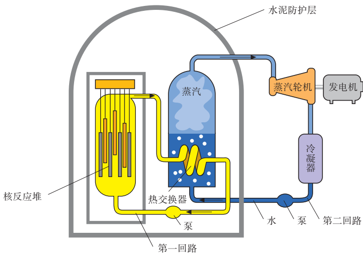
图 9.15 核电站示意图
