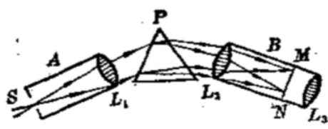
图 6.18 分光镜构造原理示意图
