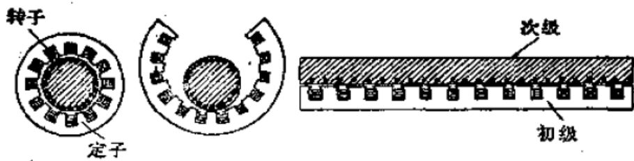
图 3.58 由旋转电机到直线电机
