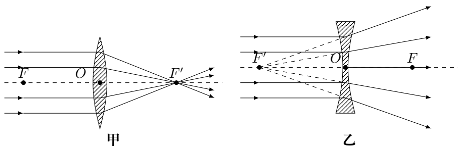
图 5.36
