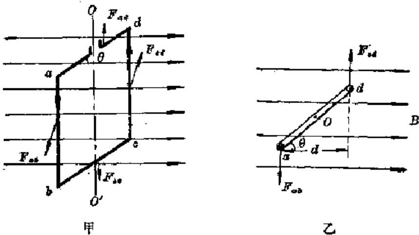
图 1.30 磁场对通电线圈的作用
