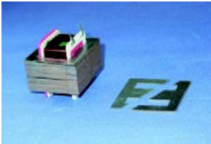
图 2.31 用硅钢片做变压器的铁芯
