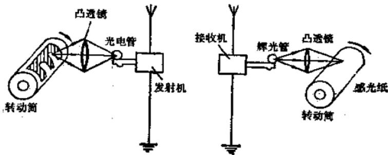
图 4.21 无线电传真示意图
