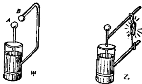
图 4.16 电谐振
