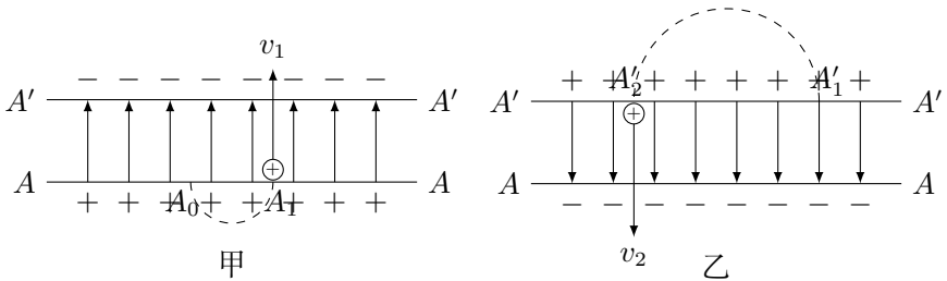
图 1.40 甲：粒子运动到 A_1 时被电场加速。乙：经过半周期，粒子运动到 A_2' ，电场改变了方向，粒子又被电场加速。
