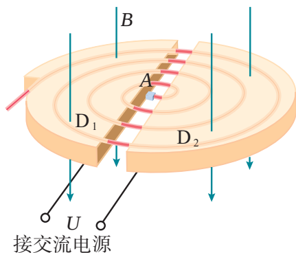
图 1.41 回旋加速器的 D 形盒
