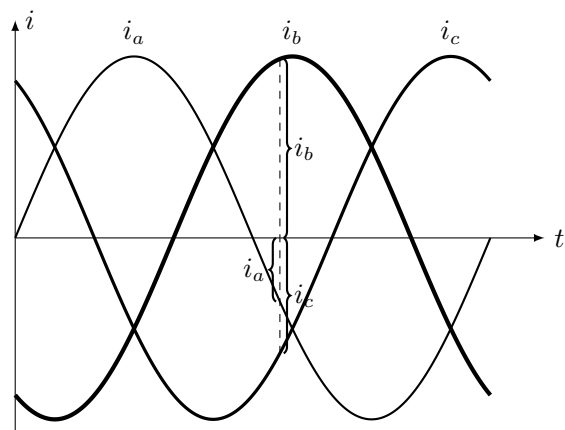
图 3.49 三相负载相同时的电流
