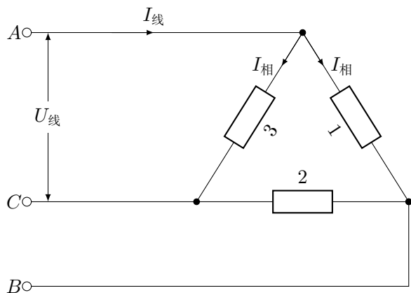
图 3.52 负载的三角形连接
