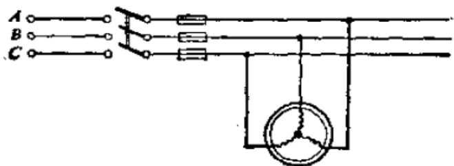
图 3.51 电动机定子线圈的星形连接
