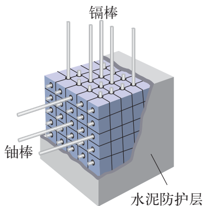
图 9.14 原子反应堆示意图
