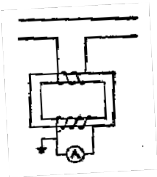
图 3.29 电流互感器
