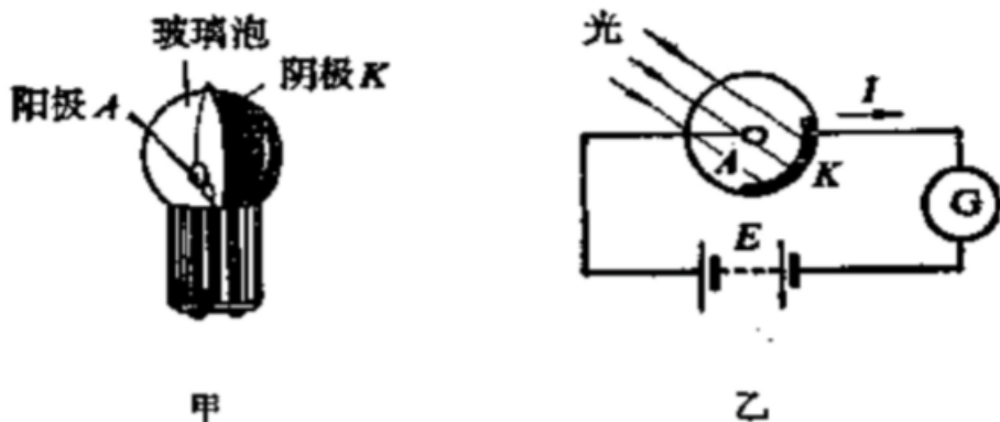
图 7.3 光电管
