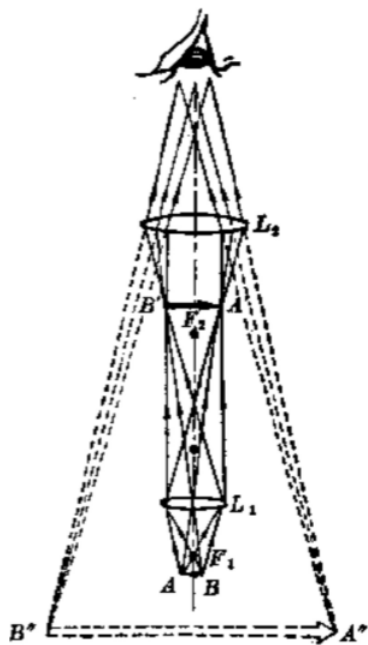
图 5.53 显微镜的成像光路图
