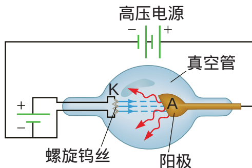
图 6.16 伦琴射线管
