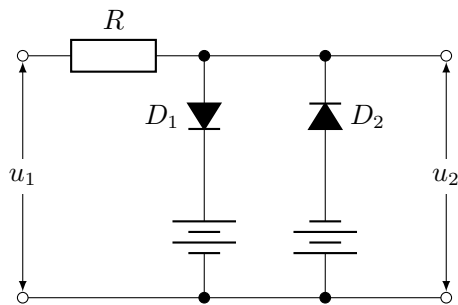
图 3.60 二极管限幅电路
