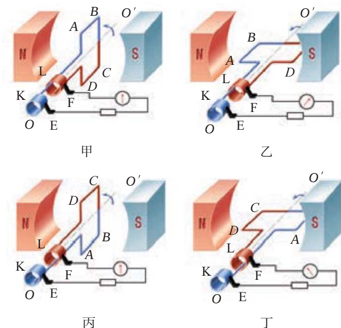
图 3.1 交流电的产生
