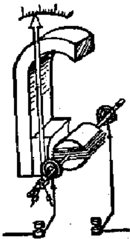
图 1.31 电流表的构造
