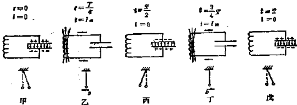
图 4.2 电磁振荡的过程
