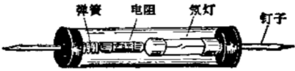
图 A.4 自制测电笔
