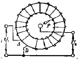
图 3.27 调压变压器
