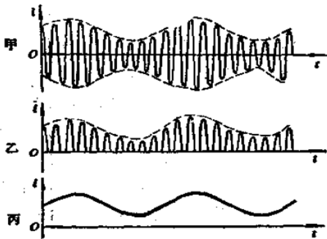
图 4.19 检波的作用
