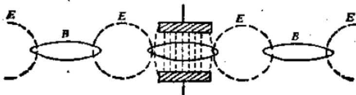
图 4.6 电磁波传播过程的示意图
