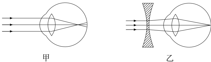
图 5.50 近视眼及其矫正方法
