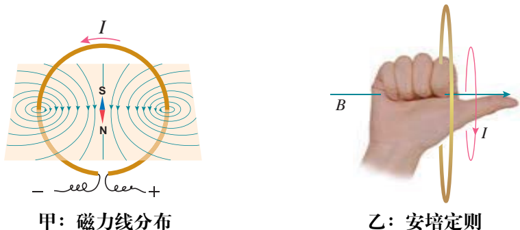
图 1.7 环形电流的磁场
