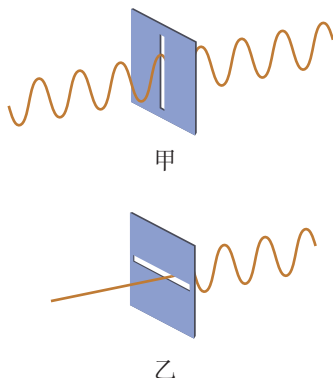
图 6.11 横波的偏振
