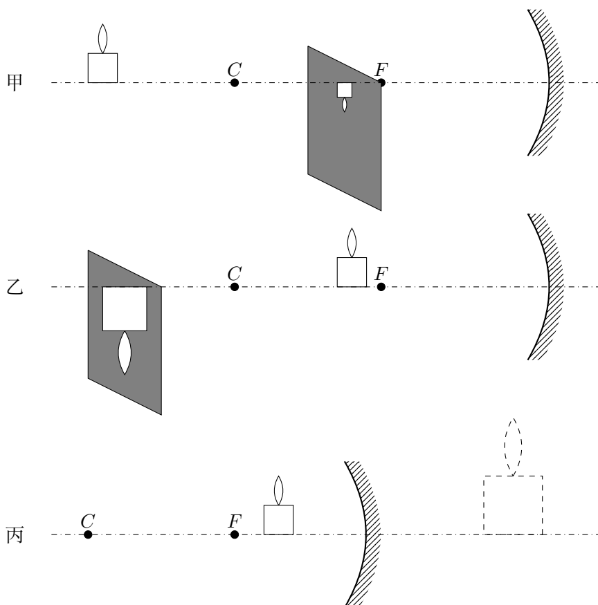
图 5.16 凹镜成像
