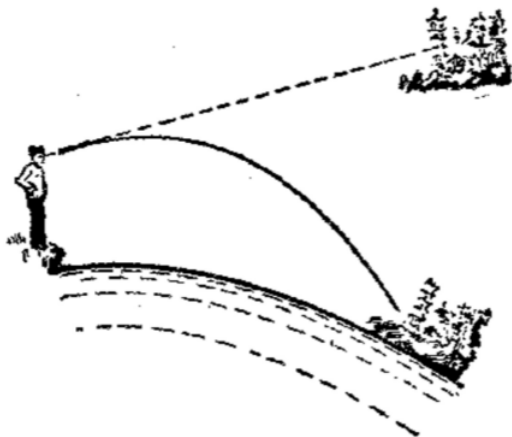
图 5.27 海市蜃楼
