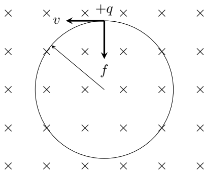
图 1.36 带电粒子的圆周运动
