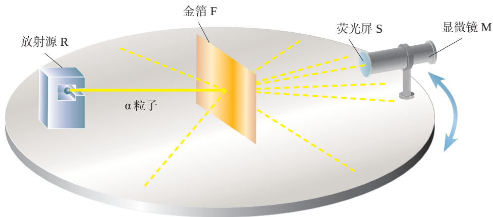
图 8.2 \alpha 粒子散射实验装置示意图
