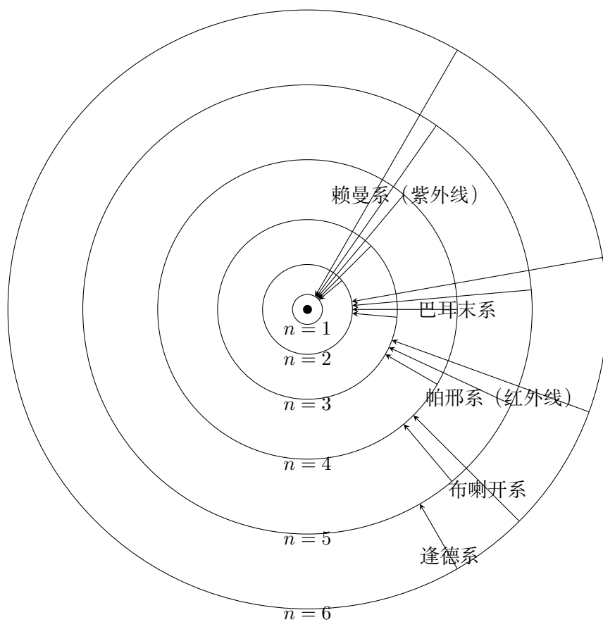
图 8.5 氢原子的轨道图
