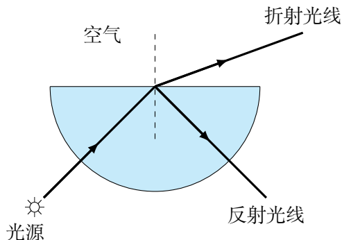
图 5.23 观察全反射现象
