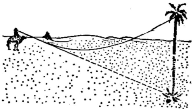
图 5.28 沙漠里的海市蜃楼
