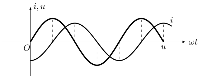
图 3.21 电感对交流电相位的影响
