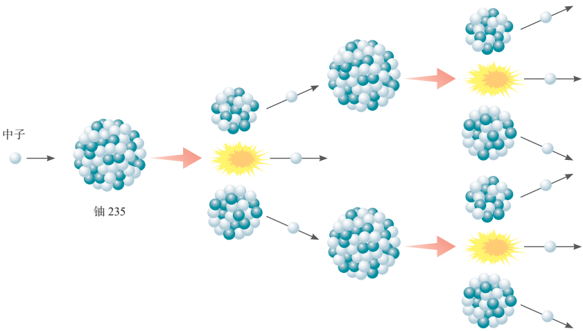
图 9.13 链式反应
