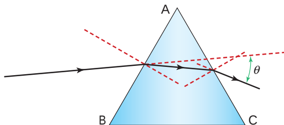
图 5.31 光线通过棱镜后, 向底面偏折
