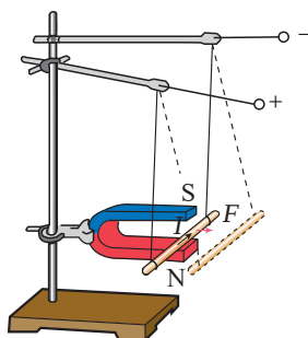
图 1.2 磁场对电流发生作用
