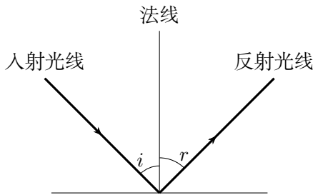
图 5.7 光的反射
