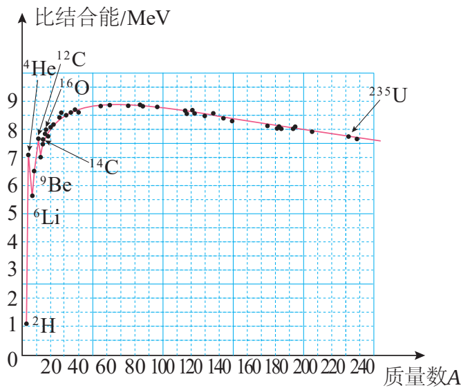
图 9.11 平均结合能曲线
