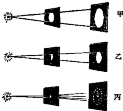
图 6.7 光通过小圆孔的衍射
