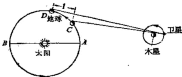
图 5.4 罗默用天文观测的方法测定光速的示意图. 设卫星第一次食毕, 地球在 C 点, 卫星绕木星公转一周, 第二次食毕, 地球在 D 点, 因此光要多传播一段距离 l 才能到达地球.
