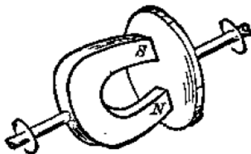
图 2.34 电磁驱动
