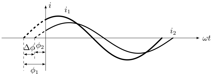
图 3.8 图中的 i_1 = I_m \sin(\omega t + \phi_1) , i_2 = I'_m \sin(\omega t + \phi_2)
