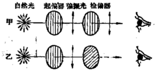
图 6.13 光的偏振
