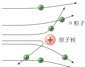
图 8.3 \alpha 粒子十分接近原子核时才会发生大角度偏转
