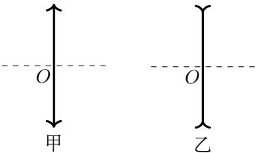
图 5.41 透镜的符号 甲：凸透镜；乙：凹透镜
