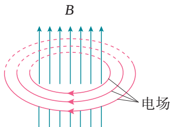
图 4.4 变化的磁场产生电场 (磁场增强时)
