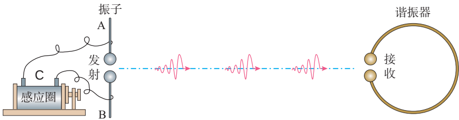
图 4.9 赫兹实验
