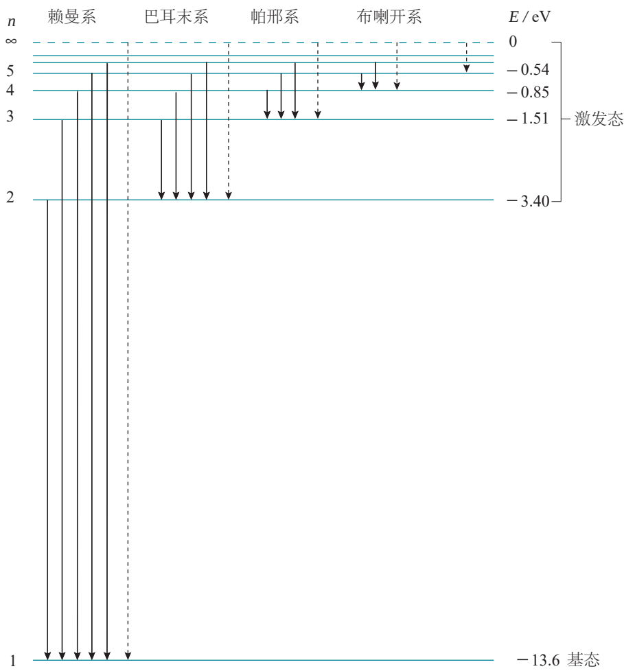
图 8.4 氢原子的能级图
