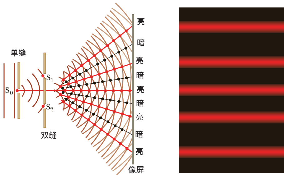
图 6.2 双缝干涉
