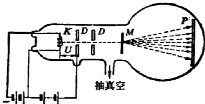
图 7.5 电子衍射实验示意图
