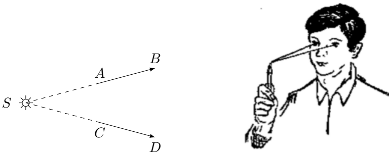
图 5.2 利用光线确定物体的位置 图 5.3 眼睛根据光的直线传播确定物体的位置
