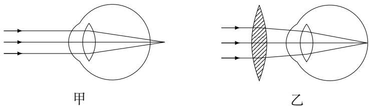
图 5.51 远视眼及其矫正方法
