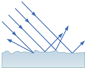
图 5.9 漫反射
