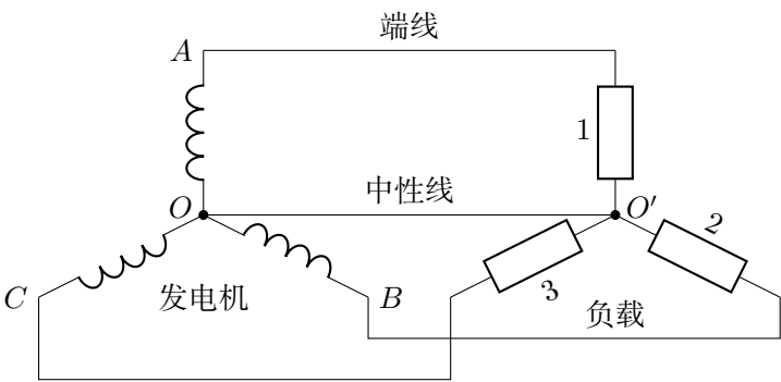
图 3.45 三相四线制
