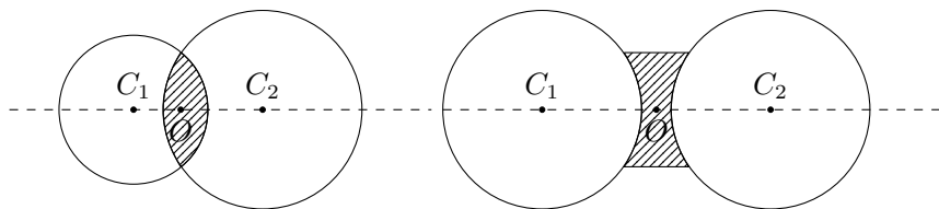
图 5.35 透镜的主轴
