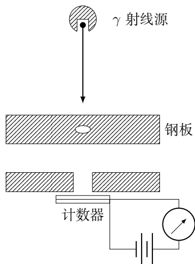
图 9.9 \gamma 射线探伤的示意图
