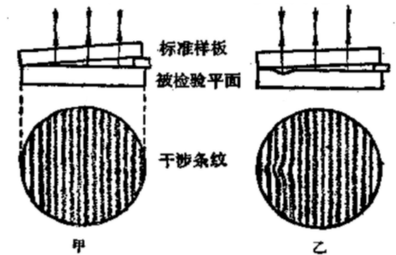
图 6.5 用干涉法检查表面
