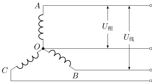
图 3.47 电源的星形连接
