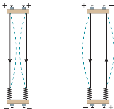
图 1.3 电流之间通过磁场发生相互作用
