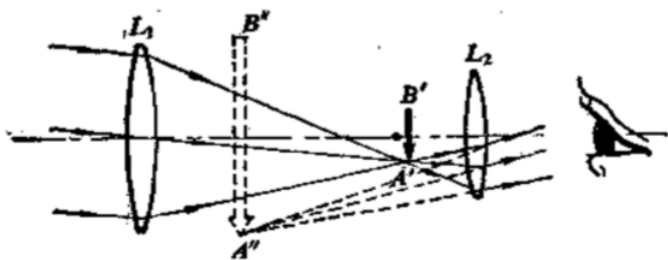
图 5.54 开普勒望远镜原理图
